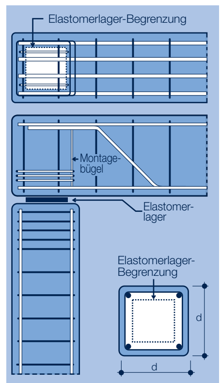
Bild 10: Methode B: Die Querschnittsbewehrung wird von einer den Bereich der Lagerfläche ringförmig umschließenden Bewehrung aufgenommen
