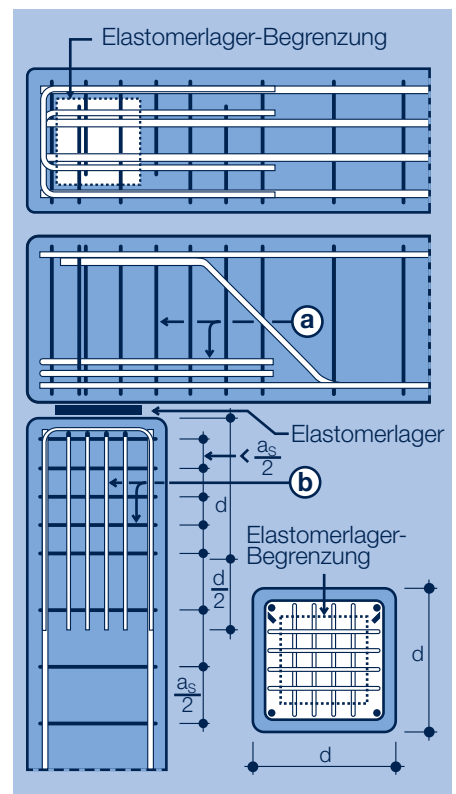
Bild 9: Methode A: Die Querschnittsbewehrung wird unmittelbar an ihrem Entstehungsort durch Bewehrung gedeckt.
