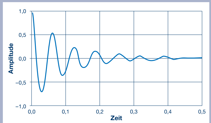
Beispiel einer CIDITAN® Ausschwingkurve
